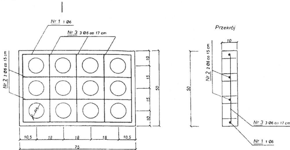
d) Płyta 0,75 × 0,50 × 0,10 m z otworami okrągłymi
